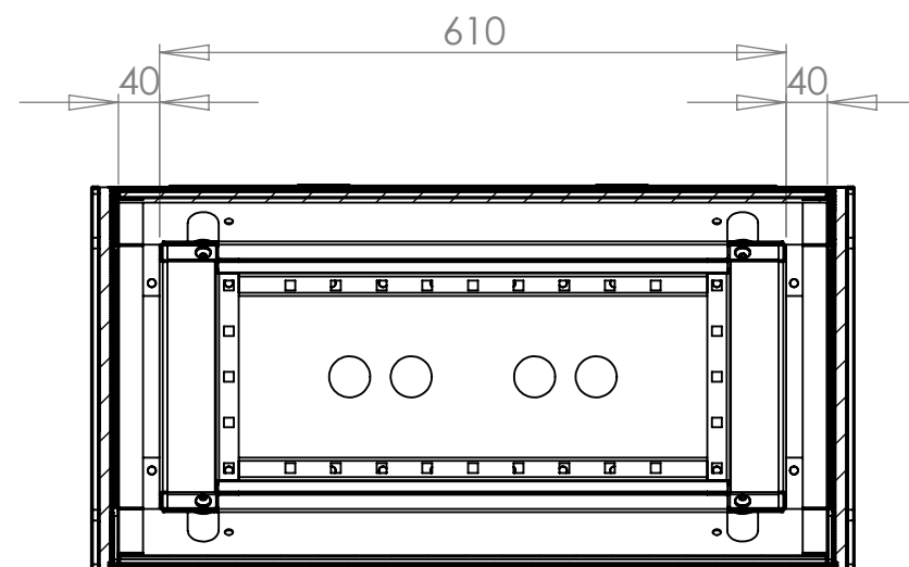
SECTION A-A SCALE 1 : 8
